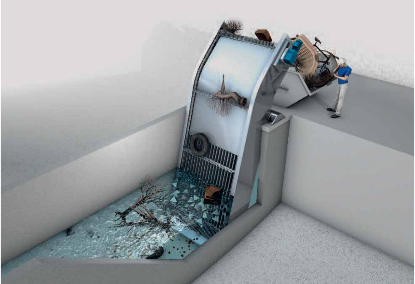
Song chắn rác thô HUBER TrashMax®
